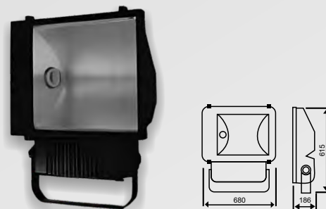
W FL E40 1000W H 491 LC
