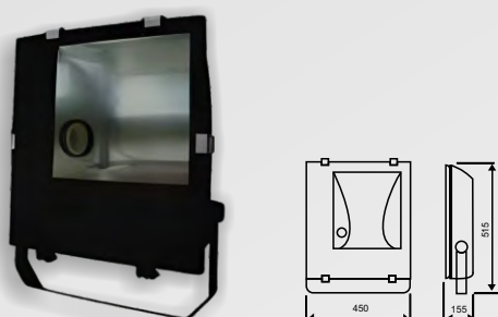
W FL E40 250-400W H 492 LC
